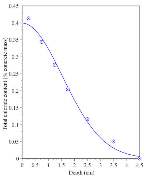
圖 3 氯離子含量與侵入深度關係示意圖
