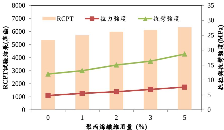
圖 11 聚丙烯纖維砂漿 91 天基本力學性質 (水灰比 0.35)
