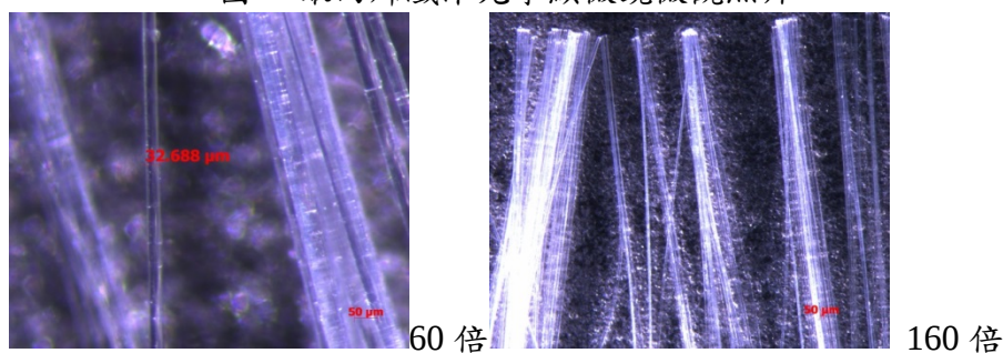
圖 8 AR 玻璃纖維光學顯微鏡微觀照片
