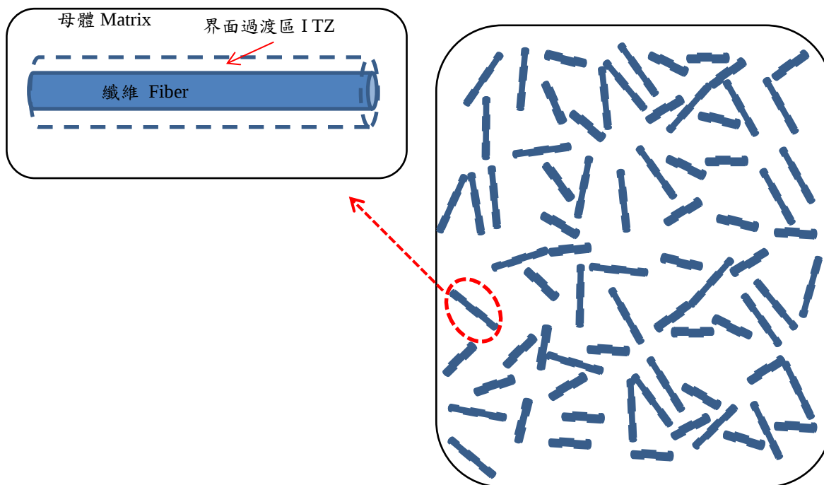
圖 5 纖維水泥複合材料示意圖
