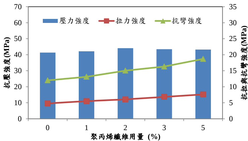
圖 10 聚丙烯纖維砂漿 91 天基本力學性質 (水灰比 0.35)
