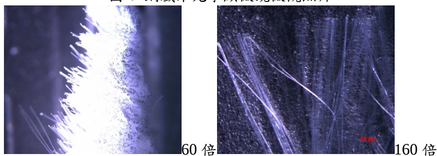
圖 7 聚丙烯纖維光學顯微鏡微觀照片
