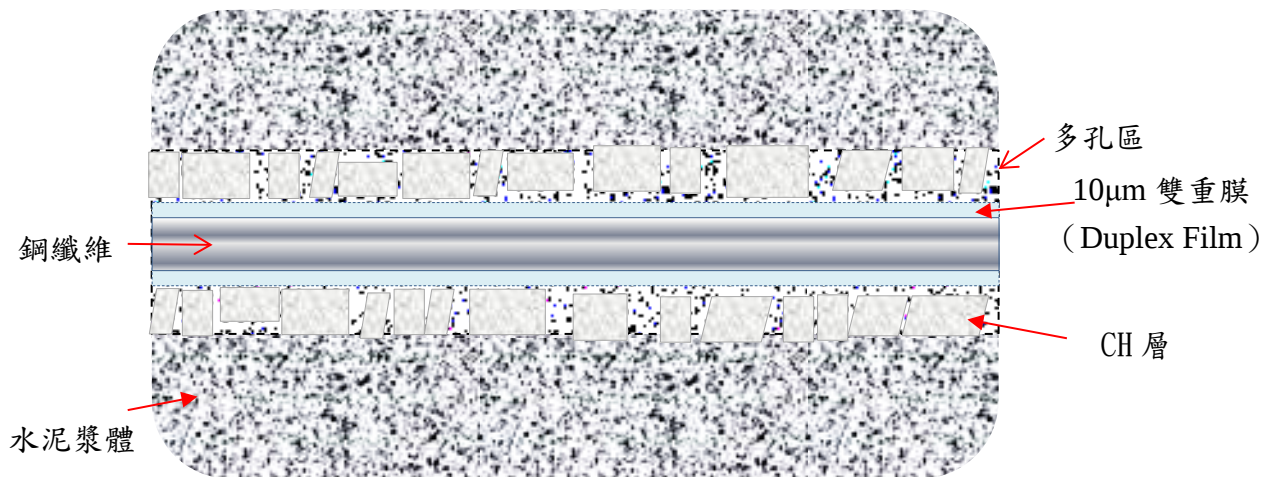
圖1 鋼纖維混凝土界面過渡區示意圖 [4]
